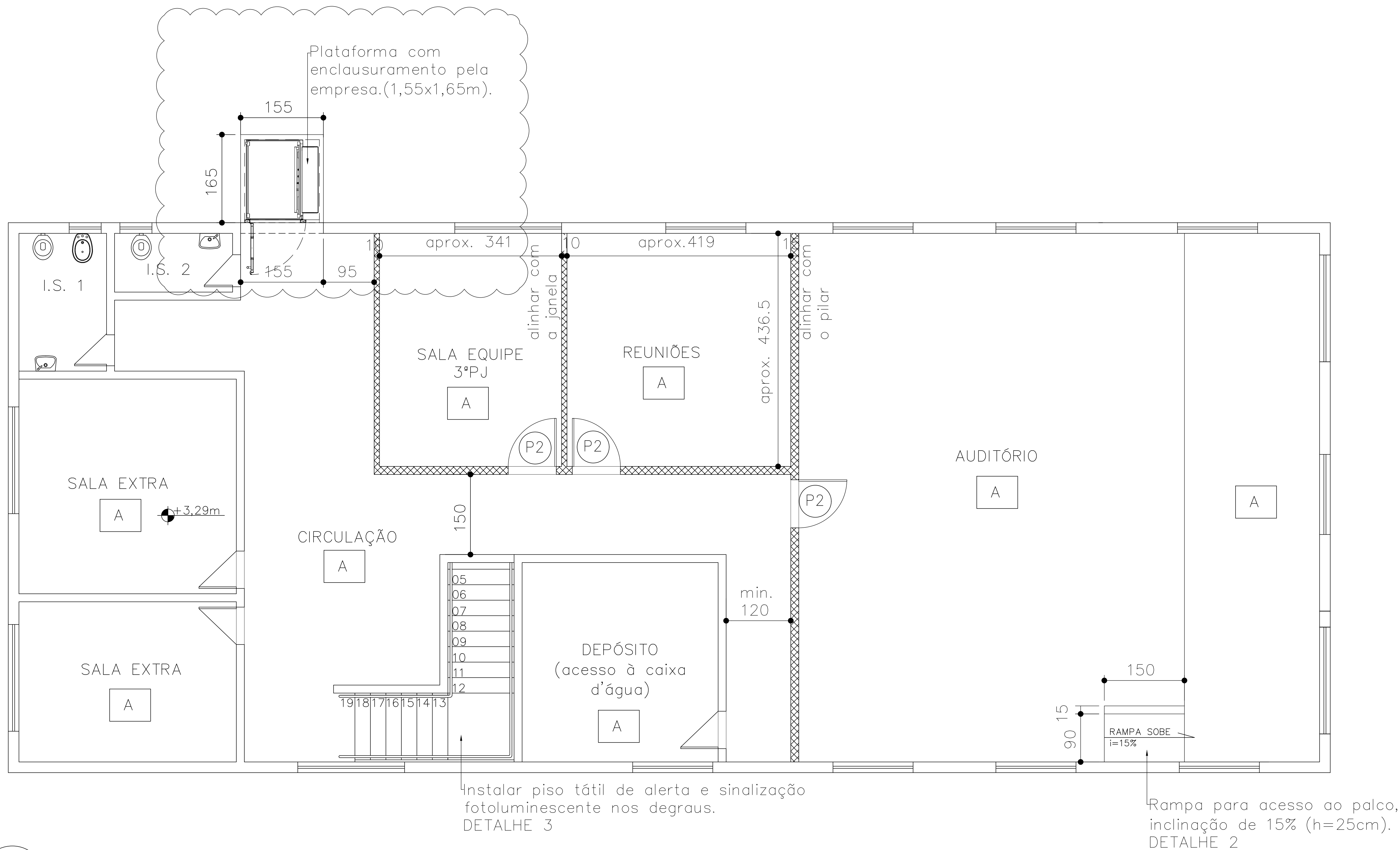
PLANTA 2º PAVTO – REFORMA ESCALA 1:100
