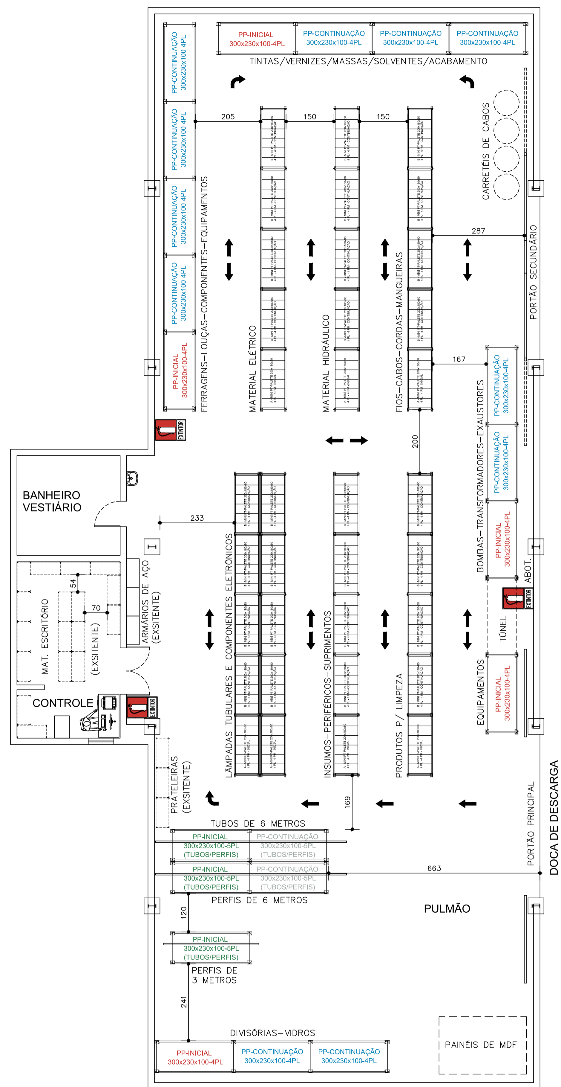
Planta Baixa / Layout Galpão do almoxarifado / suprimentos ESC 1/100
